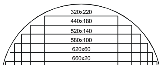
d=700 mm/0°
